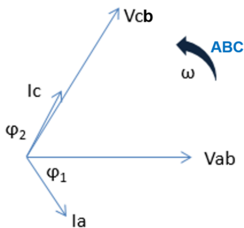
Figura 2b – Medição a dois elementos
