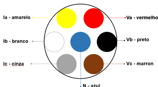
Figura 1 – Código de cores cabo controle
