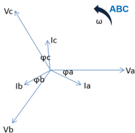
Figura 2a – Medição a três elementos
